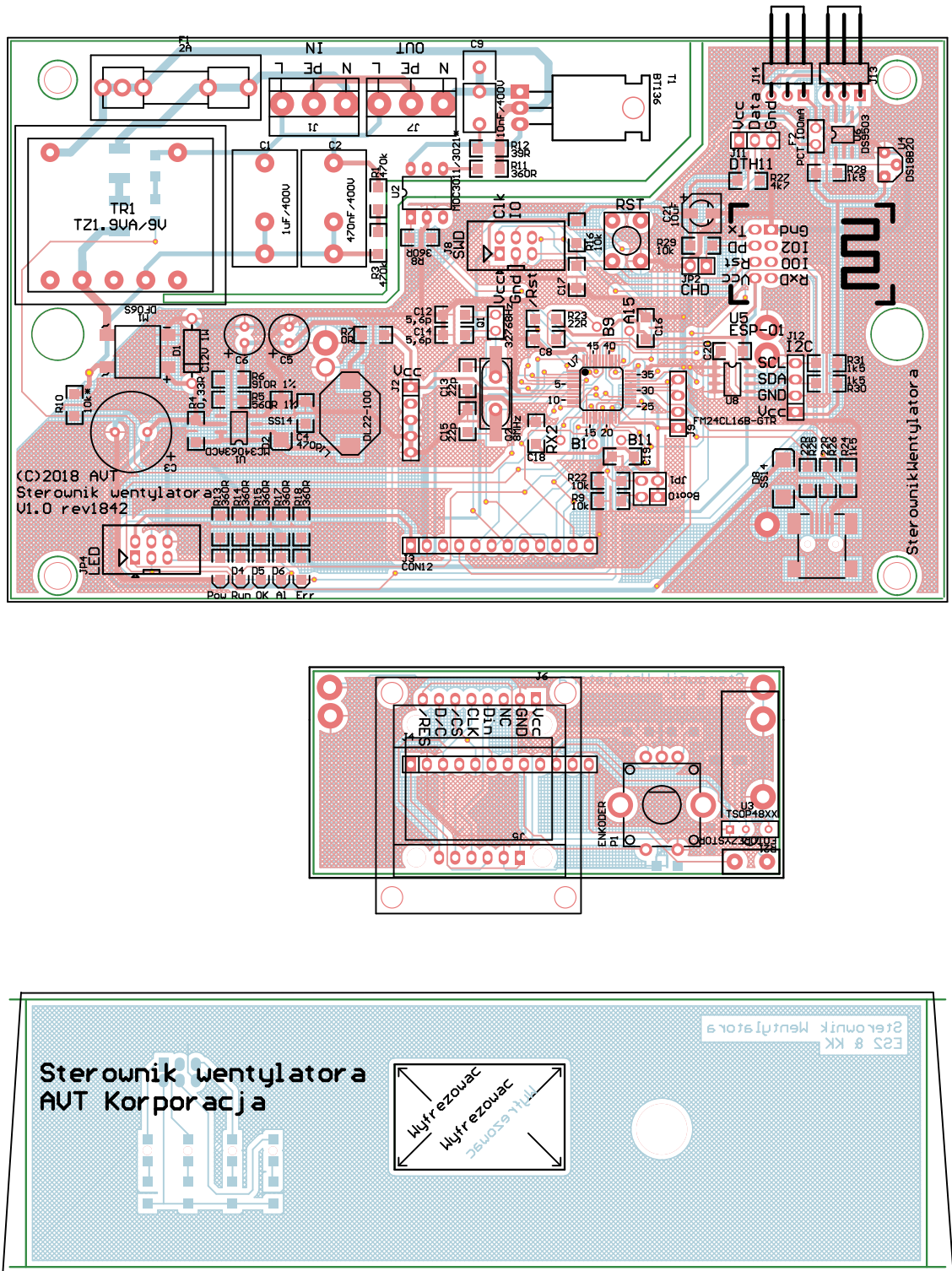
Rysunek 2. Schematy płytek wraz z rozmieszczeniem elementów oraz rysunek płyty czołowej
