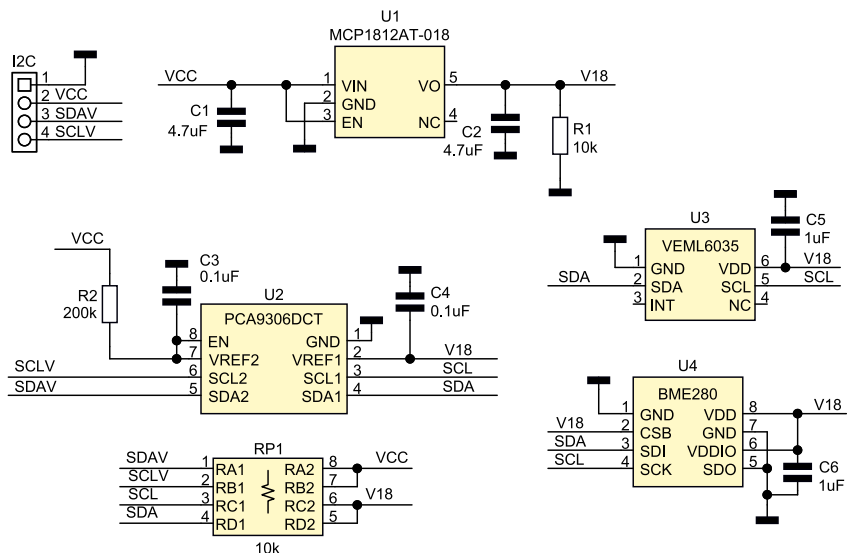
Rysunek 1. Schemat multisensora
