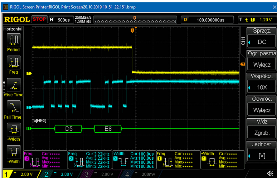
Rysunek 2. Kierunek transmisji RS485 jest zmieniany po wystaniu znaku, co pokazuje oscylogram
