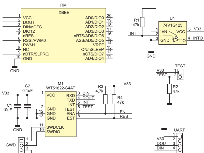
Rysunek 1. Schemat elektryczny układu
