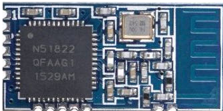
Fotografia 1. Moduł WT51822-S4AT (za notą Wireless-tag)
