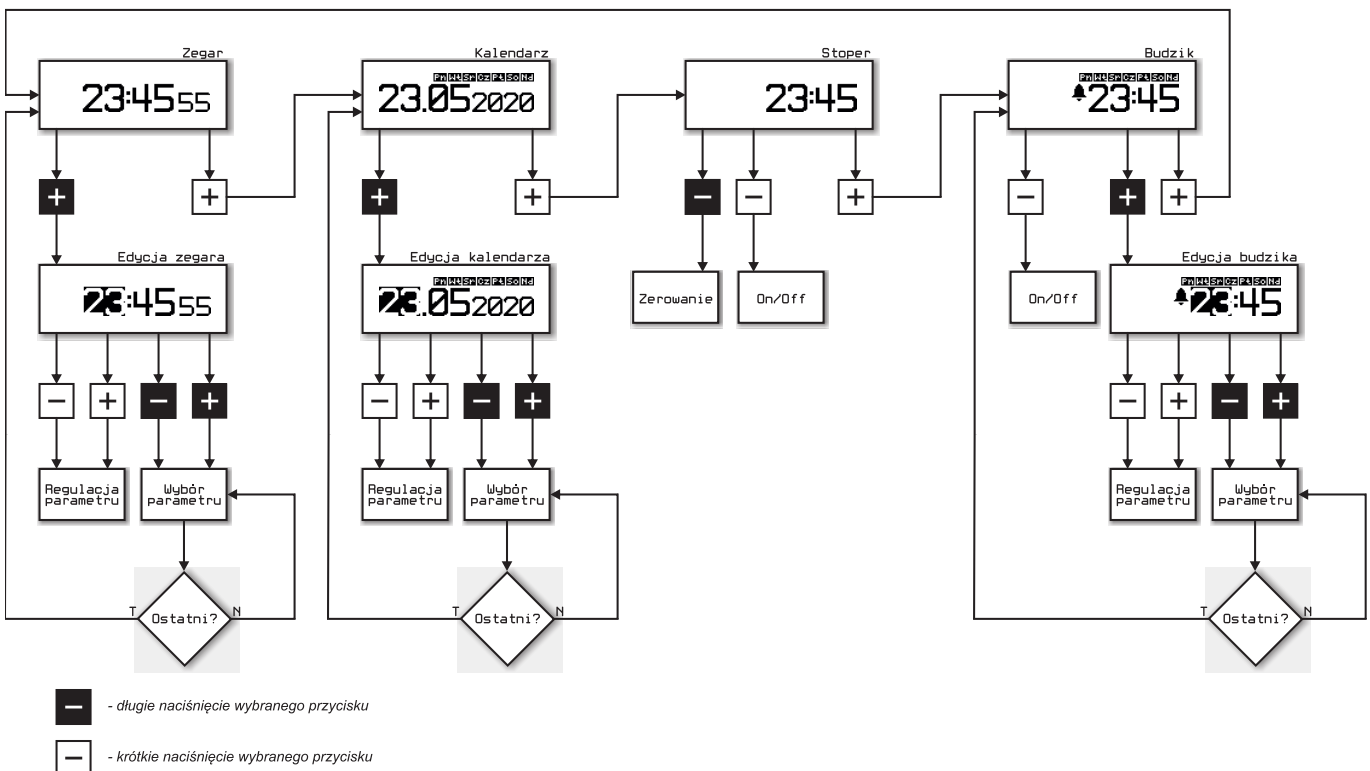
Rysunek 6. Diagram obrazujący sposób obsługi urządzenia µClock (w tym funkcjonalność przycisków funkcyjnych)
