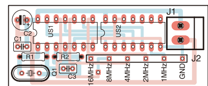
Rysunek 2. Schemat montażowy generatora sygnału TTL
