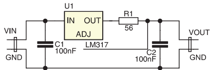
Rysunek 1. Schemat ideowy zasilacza do modułów laserowych
