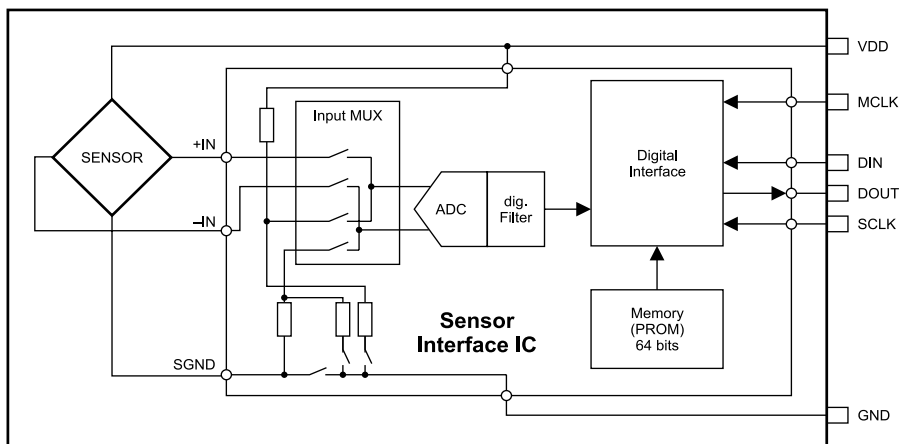
Rysunek 4. Schemat blokowy czujnika ciśnienia atmosferycznego MS5534A
