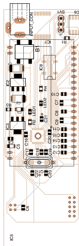
Rysunek 8. Schemat montażowy miernika parametrów środowiskowych
