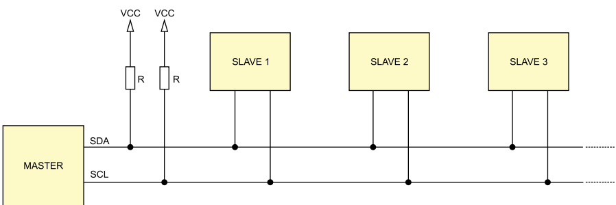
Rysunek 6. Magistrala I 2 C
