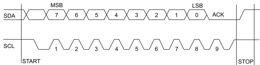
Rys. 7. Ramka danych w standardzie I 2 C
