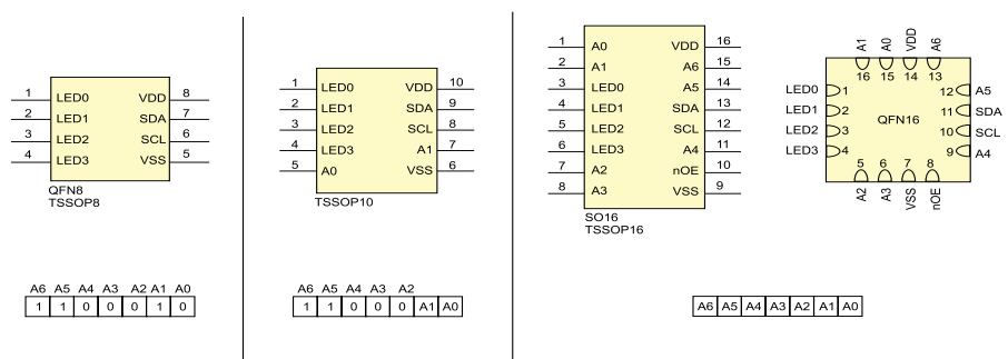
Rysunek 2. Konfigurowanie adresu układu PCA9633 w zależności od wersji obudowy
