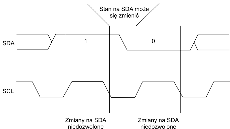
Rys. 8. Kodowanie wartości logicznych
