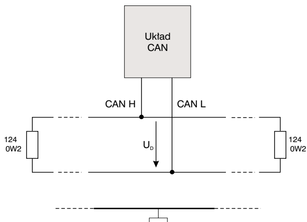
Rys. 3. Dotychczasanie elementu (stacji) do magistrali CAN.
