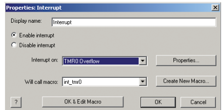
Rys. 4. Odblokowanie i konfiguracja przerwania od przepełnienia TMR0
