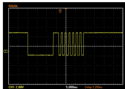
Rys. 3. Oscylogram komendy zwalniania migawki Pentax
