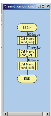
Rys. 18. Makro komendy aparatu Canon
