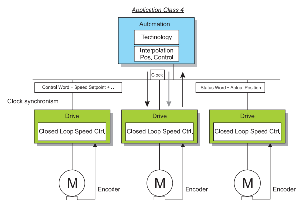
Rys. 5. PROFIdrive, pozycjonowanie z centralną interpolacją i pozycjonowaniem
