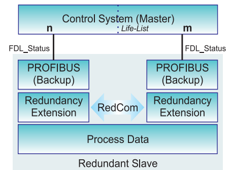
Rys. 4. Redundancja stacji slave w sieci Profibus
