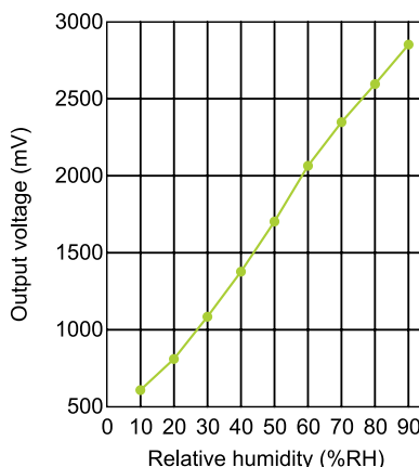
Rysunek 2. Zależność napięcia wyjściowego czujnika HS-230A od wilgotności względnej ( V_{cc}=5V )
