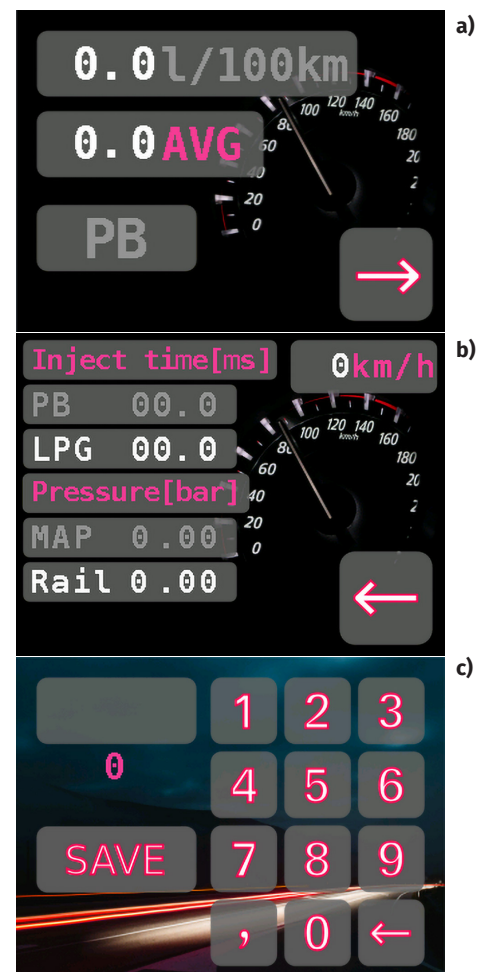
Fotografia 4. Komunikaty na wyświetlaczu: a) strona główna spalanie chwilowe i średnie, b) podgląd podstawowych parametrów pracy silnika, c) strona kalibracji – można wprowadzić ilość zatankowanego paliwa
