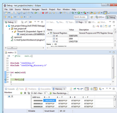
Rysunek 7 Widok perspektywy Debug w środowisku AC6 System Workbench
