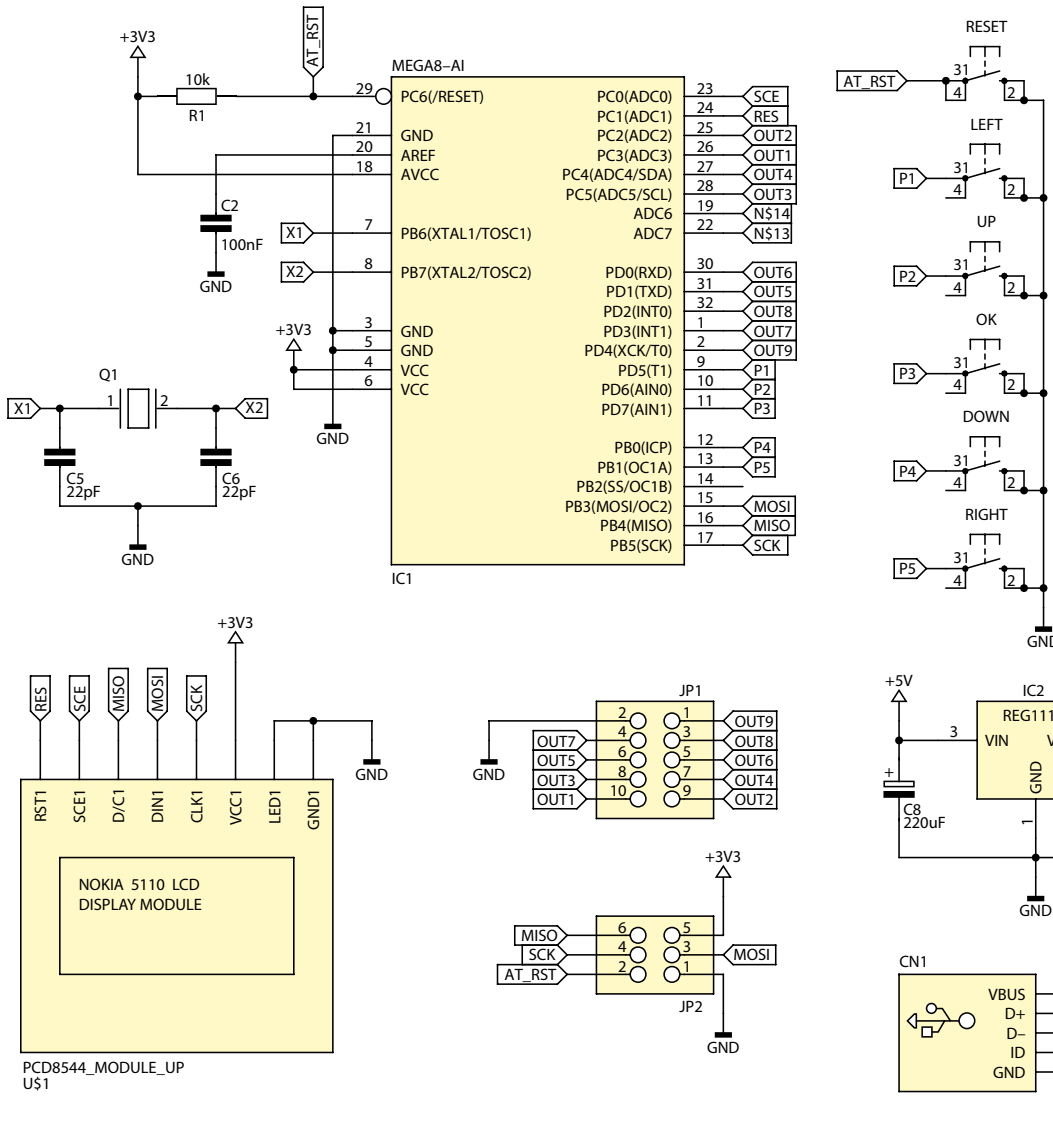
Rysunek 1. Schemat ideowy gry elektronicznej „Snake”
