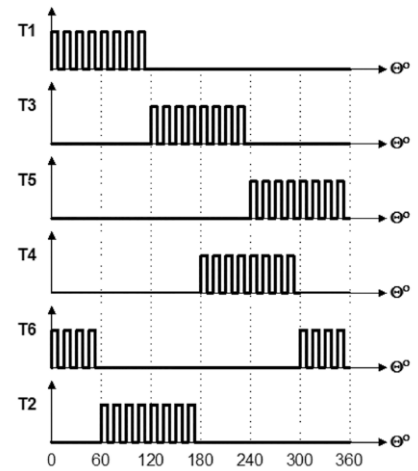
Rysunek 11. Sekwencja przełączeń zaworów komutatora dla sterowania bipolarnego
