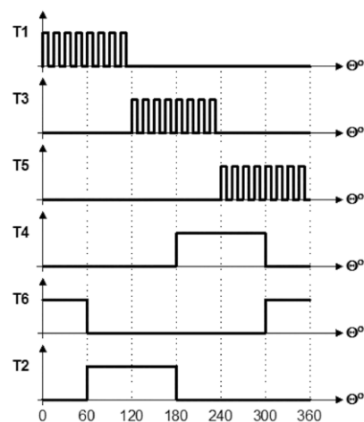
Rysunek 3. Sekwencja przełączeń zaworów komutatora dla strategii sterowania C120Q+
