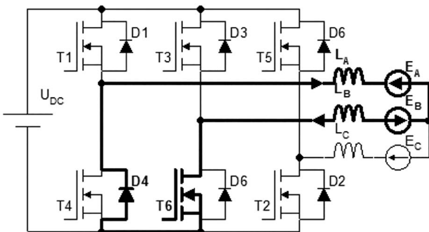
Rysunek 8. Schemat zastępczy silnika przy strategii typu C120Q+ (tranzystor regulujący T1 wyłączony)
