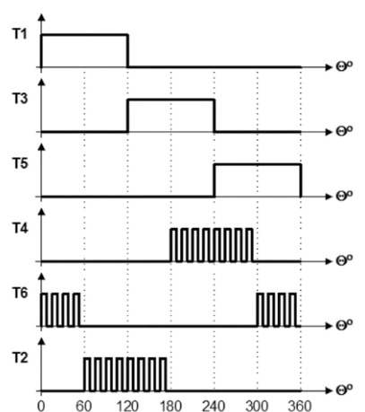
Rysunek 4. Sekwencja przełączeń zaworów komutatora dla strategii sterowania C120Q-
