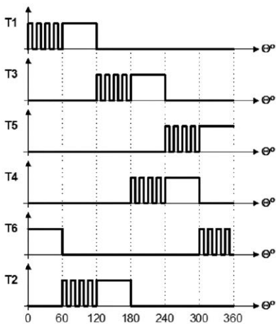
Rysunek 5. Sekwencja przełączeń zaworów komutatora dla strategii sterowania C60Q+
