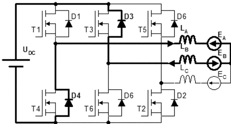
Rysunek 12. Schemat zastępczy silnika dla sterowania bipolarnego (tranzystory regulujące T1 oraz T6 wyłączone)
