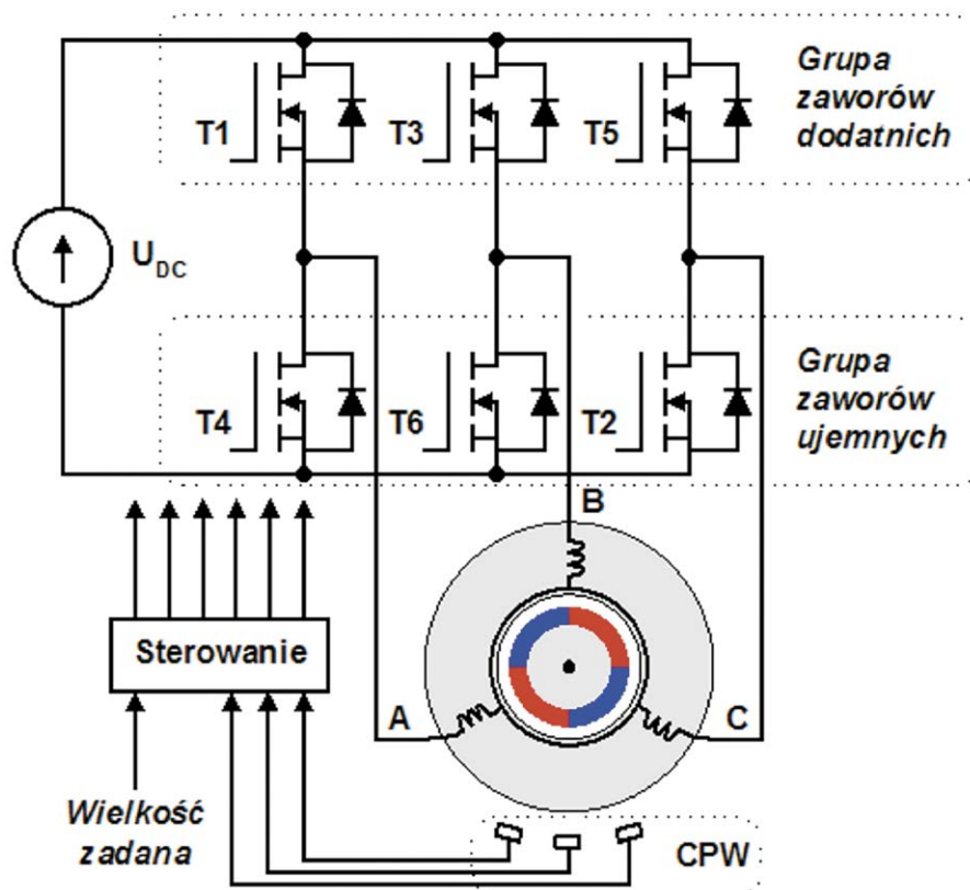
Rysunek 1. Schemat napędu z silnikiem BLDC
