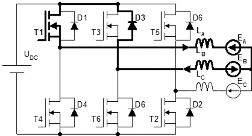
Rysunek 9. Schemat zastępczy silnika przy strategii typu C120Q- (tranzystor regulujący T6 wyłączony)
