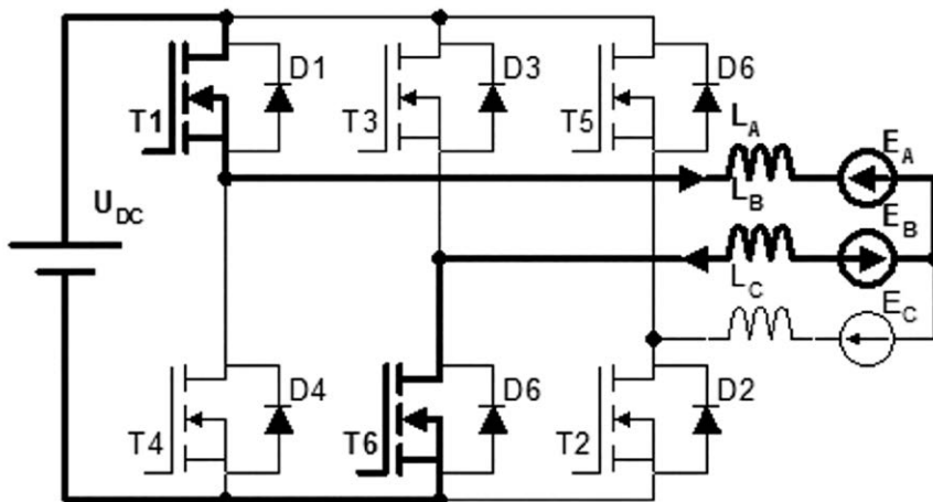
Rysunek 7. Schemat zastępczy silnika BLDC przy załączonych dwu tranzystorach
