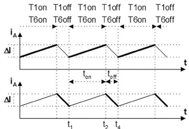
Rysunek 13. Przebieg prądu fazowego silnika przy zastosowaniu sterowania bipolarnego
