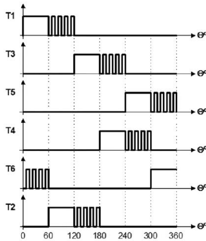
Rysunek 6. Sekwencja przełączeń zaworów komutatora dla strategii sterowania C60Q-
