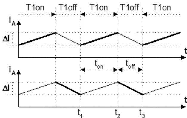
Rysunek 10. Przebieg prądu fazowego silnika dla strategii C120Q+ (w stanie ustalonym)
