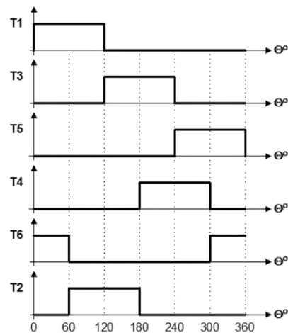
Rysunek 2. Ogólna sekwencja przełączeń zaworów komutatora elektronicznego dla klasycznych strategii sterowania silnikiem BLDC
