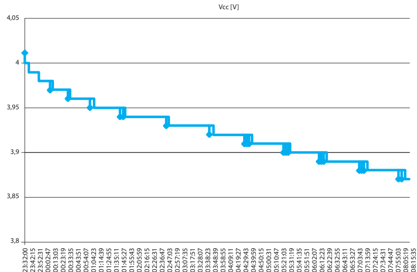
Rysunek 6. Wykres napięcia zasilania w funkcji czasu
