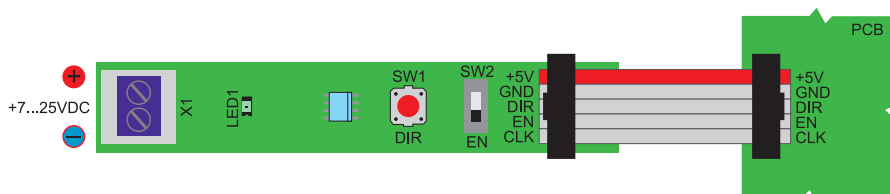
Rysunek 3. Schemat przyłączenia sterownika – wariant 1
