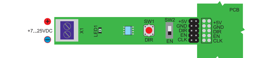
Rysunek 4. Schemat przyłączenia sterownika – wariant 2
