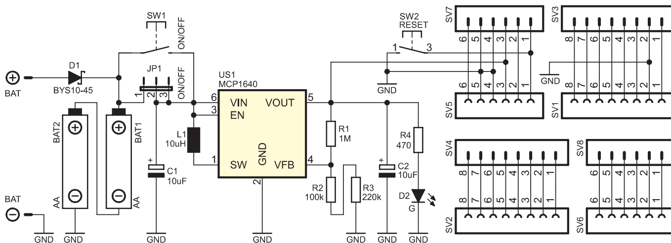
Rysunek 1. Schemat ideowy AVTduino Battery Shield
