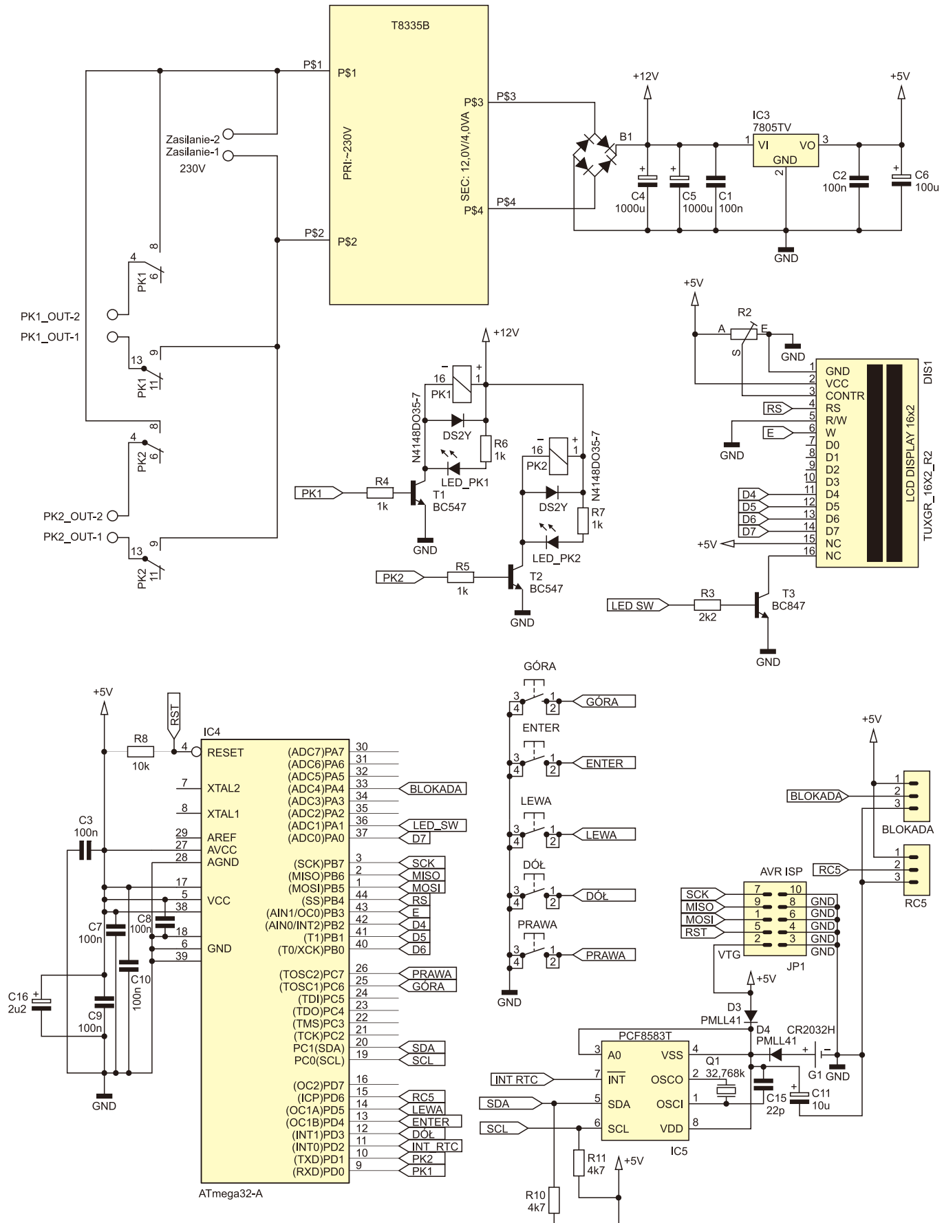
Rysunek 1. Schemat ideowy włącznika programowanego
