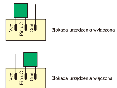
Rysunek 3. Funkcjonowanie zworki „Blokada”
