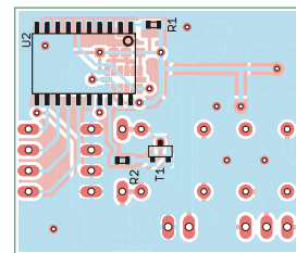
Rysunek 4. Schemat montażowy układu ASO
