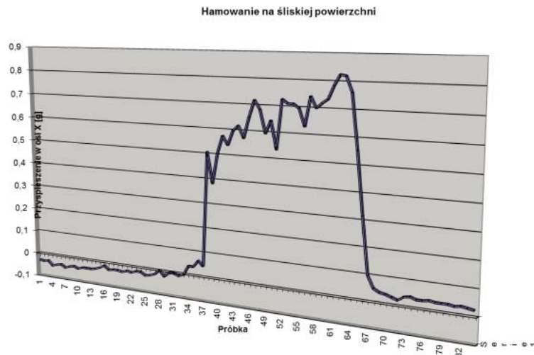
Rysunek 5. Wykres zależności przyspieszenia w funkcji czasu zarejestrowany podczas hamowania na śliskiej powierzchni
